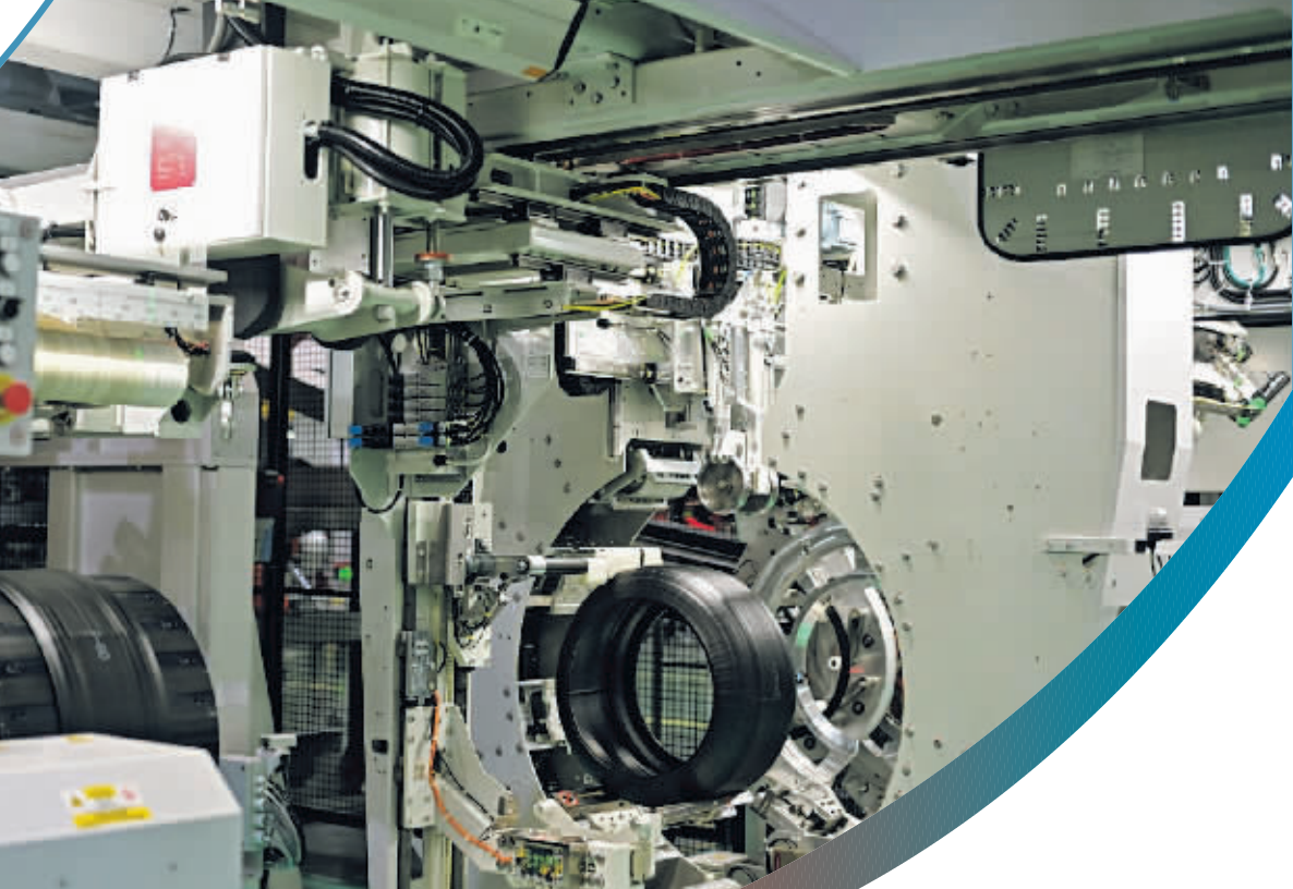
2024年7月26日拍摄的浙江杭州中策钱塘实业有限公司轮胎数字工厂车间内的自动化轮胎生产线。
