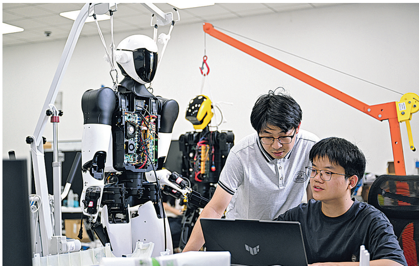
2025年5月29日,在位于湖北省武汉市的华中科技大学机械科学与工程学院,研究人员对“荆楚”人形机器人进行代码调试。 新华/传真
