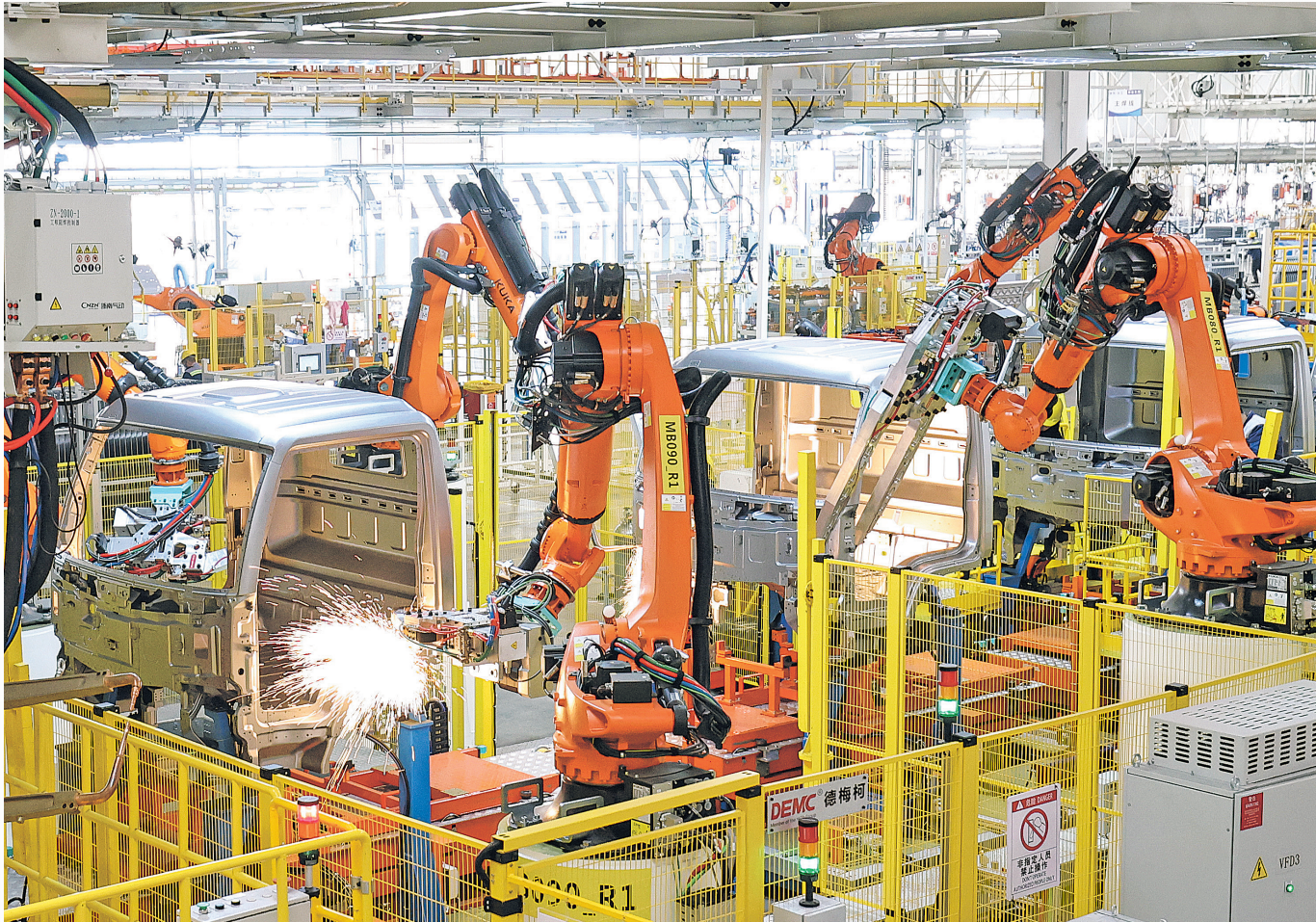
贵州长江汽车有限公司全新焊装机器人生产线。
